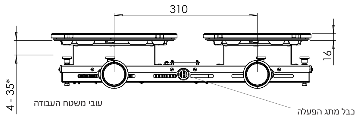
מבט חזיתי
