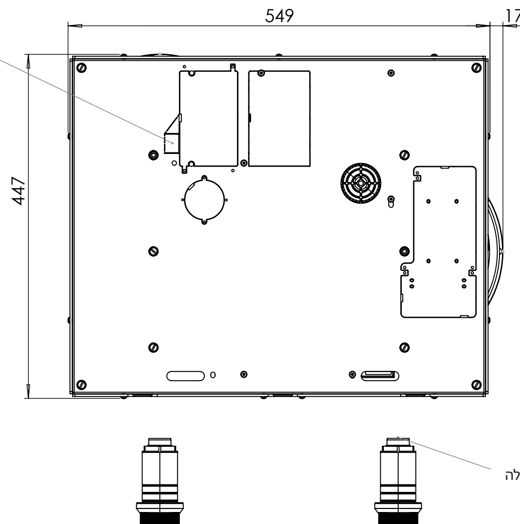
מבט תחתון
