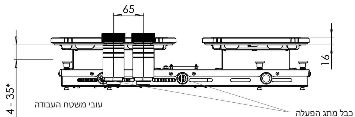
מבט חזיתי
