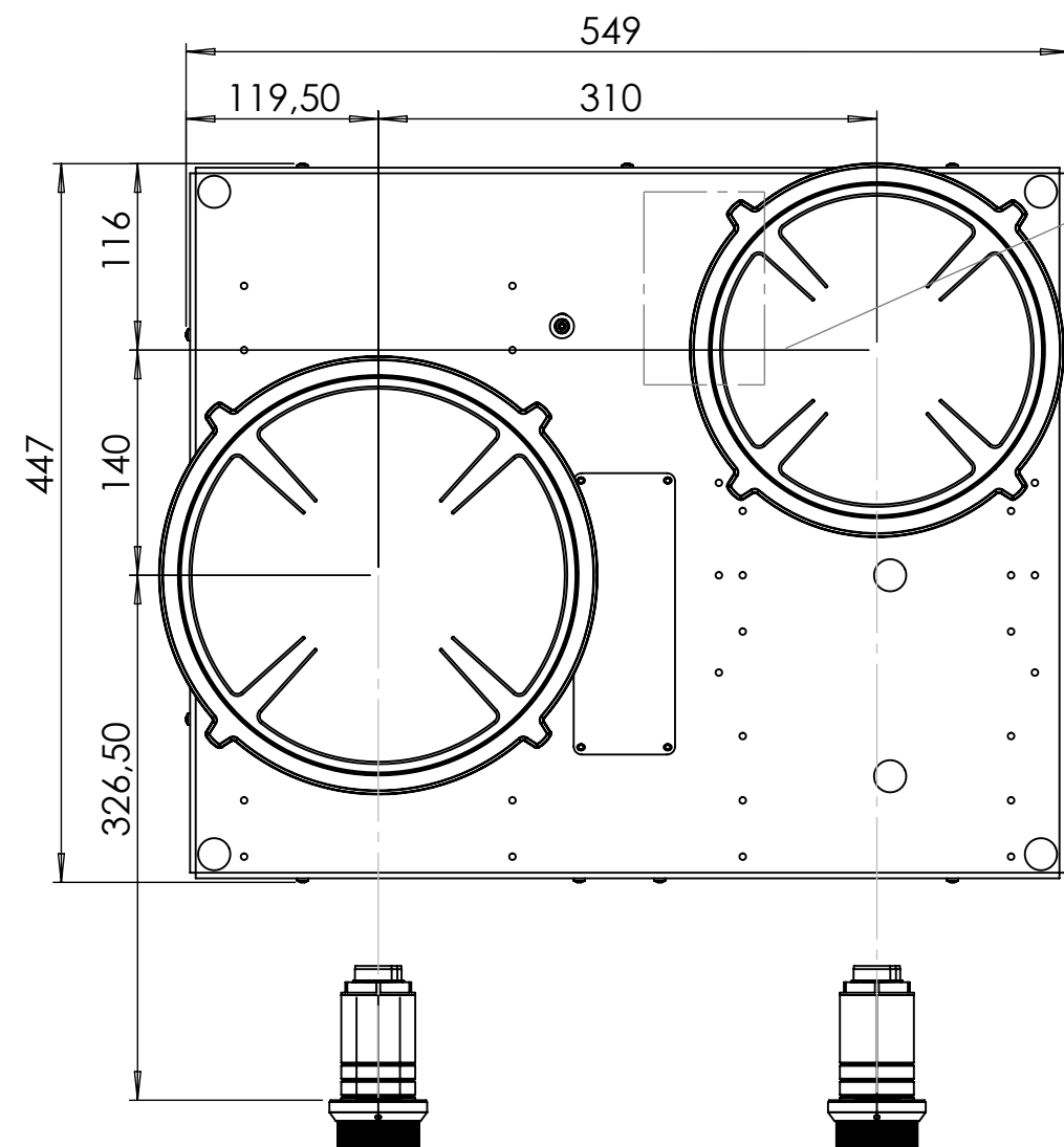
מבט עליון
