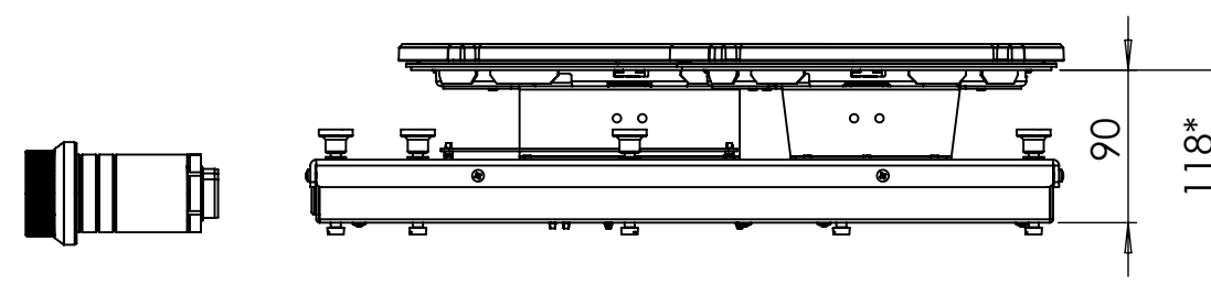
מבט צדדי
